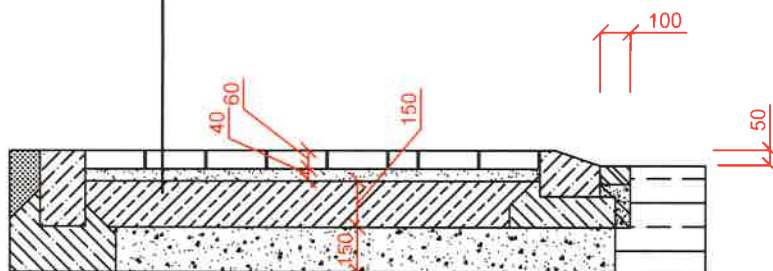
VZOROVÝ REZ CHODNÍKOM (v mieste vjazdu)
