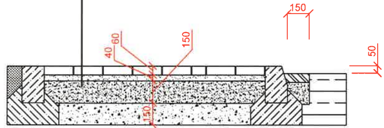
VZOROVÝ REZ CHODNÍKOM
